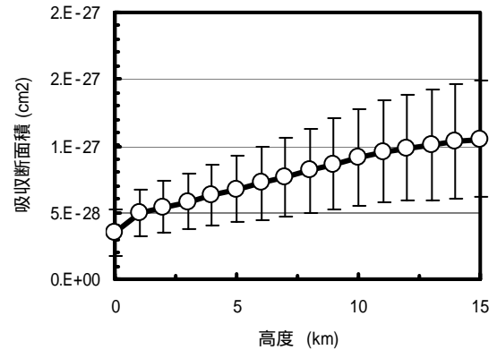
Fig. 4 高度 0km から 15km までの吸収断面積
