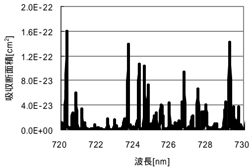
Fig. 2 波長 720nm から 730nm の吸収断面積の波長依存性
