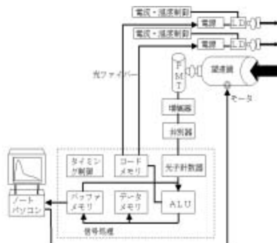
Fig. 1 RM-CW DIAL の原理図
