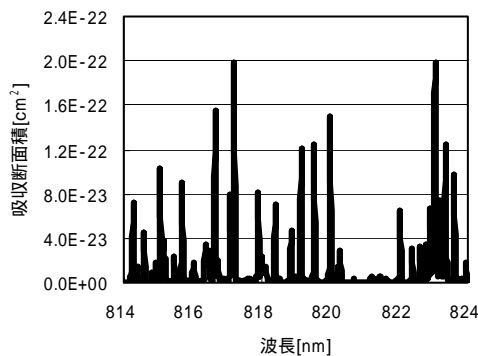
Fig. 3 波長 814nm から 824nm の吸収断面積の波長依存性
